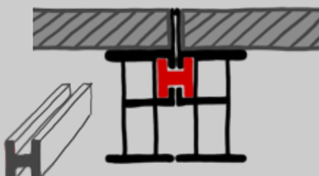
H-Profil-Verbinder
