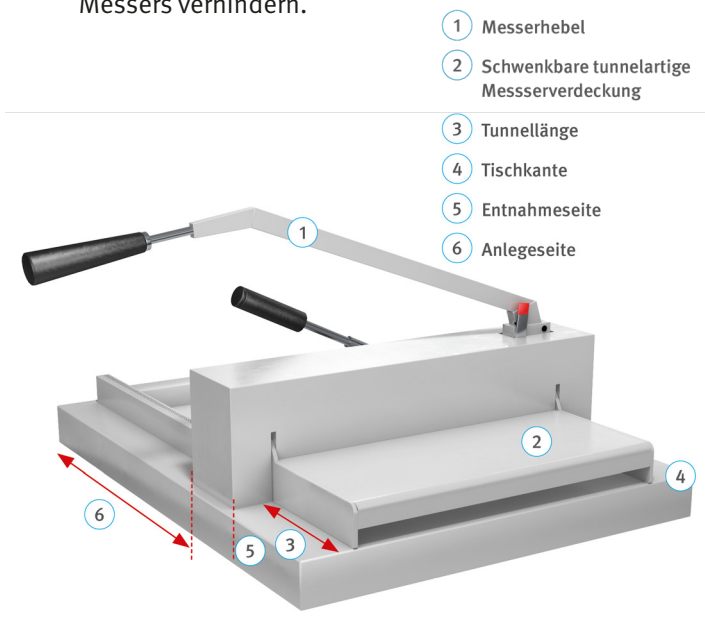
Abb. 11 Messerverdeckung auf Entnahmeseite
