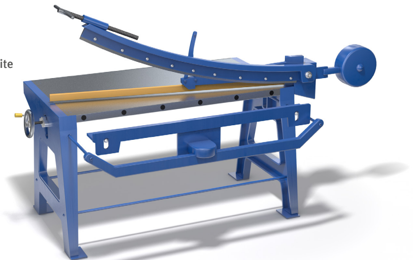
Abb. 4 Pappschere
