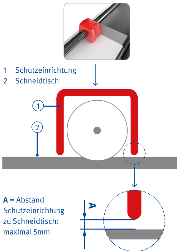
Abb. 13 Schutzeinrichtung über dem Kreismesser
