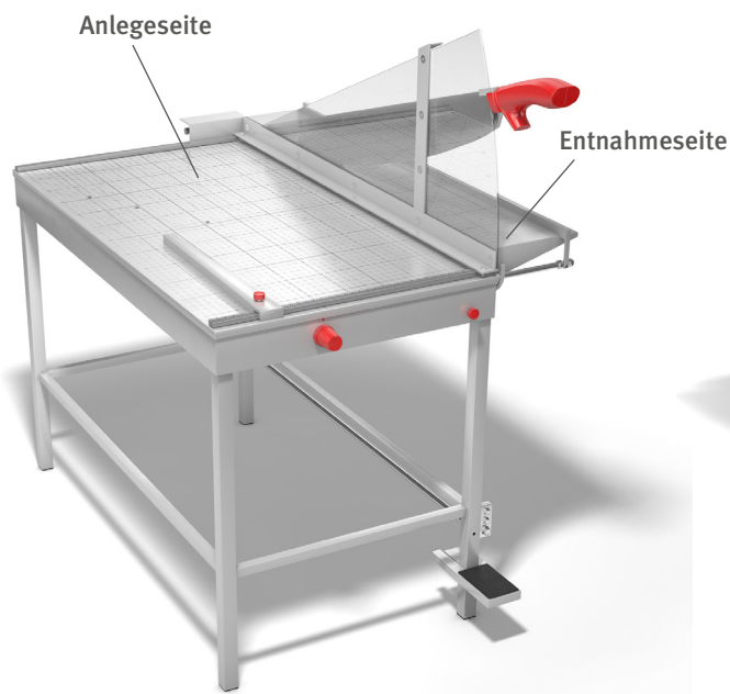
Abb. 1 Hebelschneider
