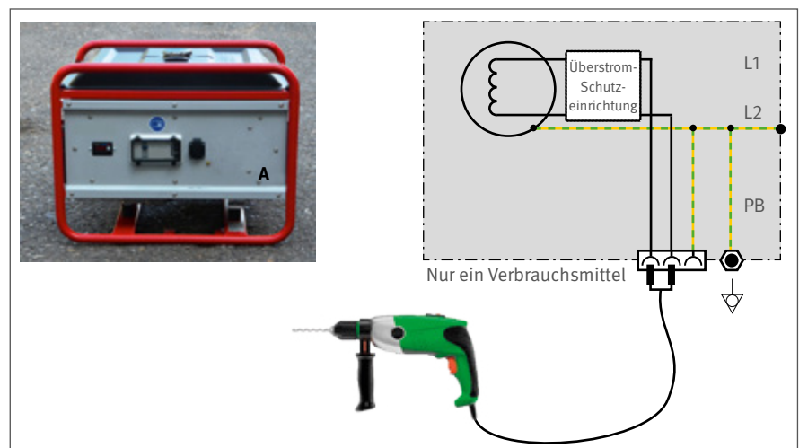
Abb. 6 Stromerzeuger ohne Erdungsanschluss mit nur einer Steckdose und nur einem angeschlossenen Verbrauchsmittel
