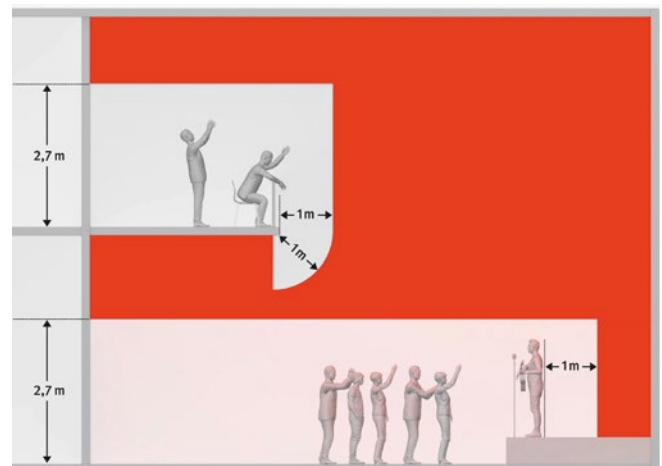
Abb. 3 Abgrenzung zwischen dem Zuschauerbereich und dem Showlaserbereich
