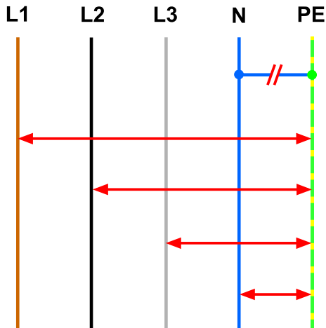
Abb. 19 Isolationswiderstandsmessung; Einzelmessung
