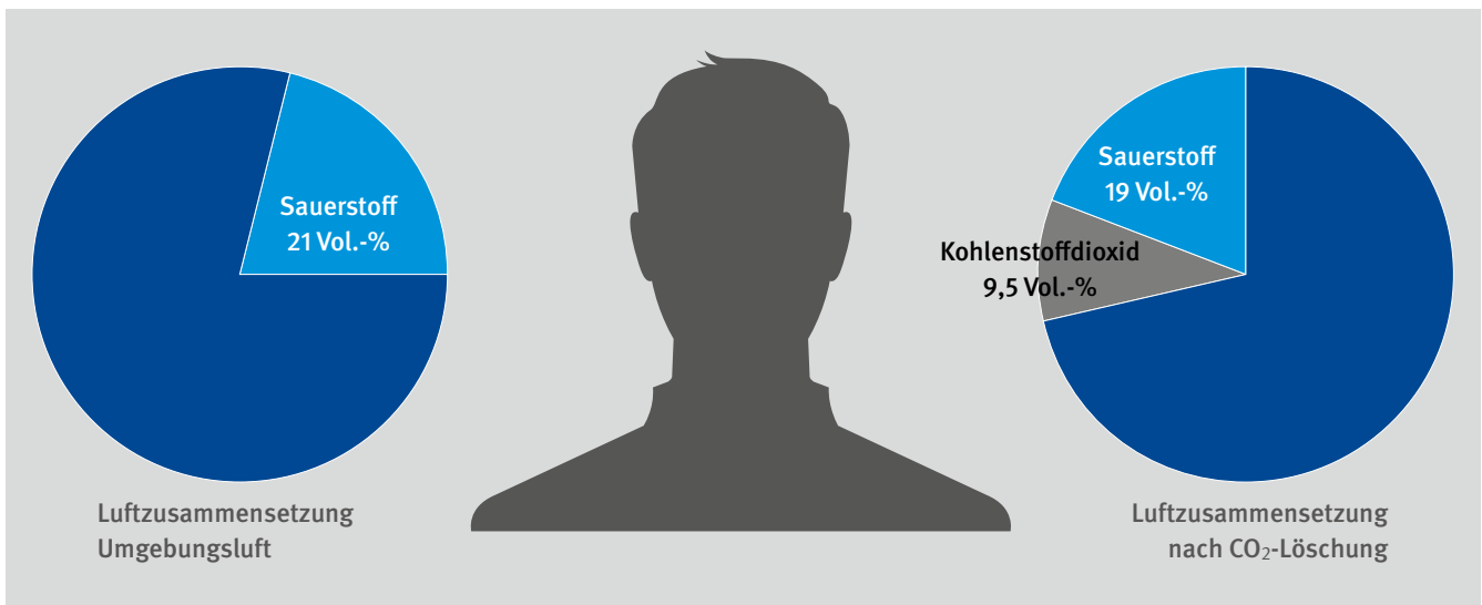
Abb. 3 Darstellung der Luftzusammensetzung in Vol.-% vor (links) und nach (rechts) eines Löschversuchs mit CO 2 , gemessen in Atemhöhe (1,65 m). Es besteht Vergiftungsgefahr durch CO 2 , obwohl der Sauerstoffgehalt mit 19 Vol.-% noch völlig ausreichend erscheint.
