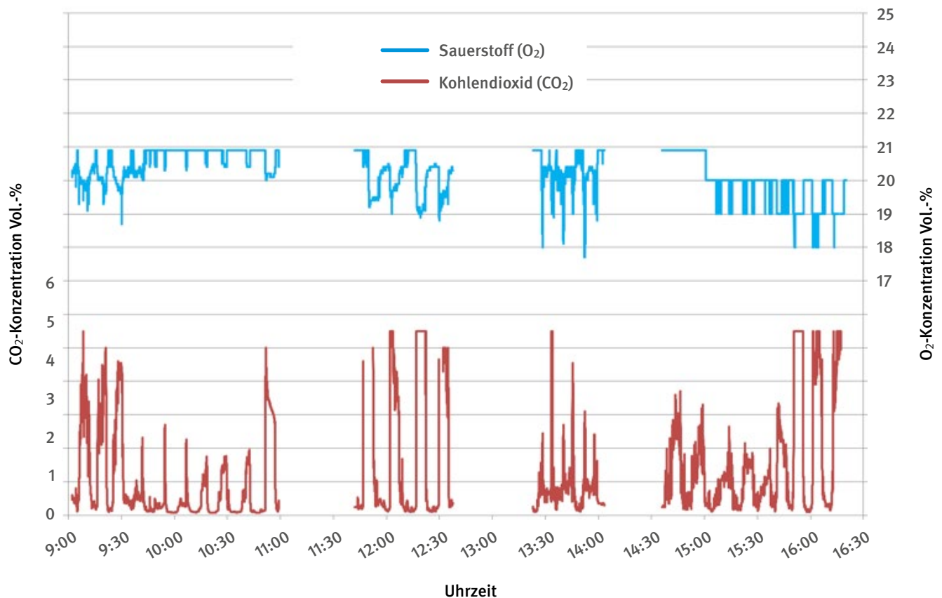
Abb. 4 Beispielhaftes Diagramm mit Messergebnissen der personengetragenen Detektion im Vergleich Kohlendioxid (CO 2 ) zu Sauerstoff (O 2 ) in der Atemluft (Quelle: IFA)
