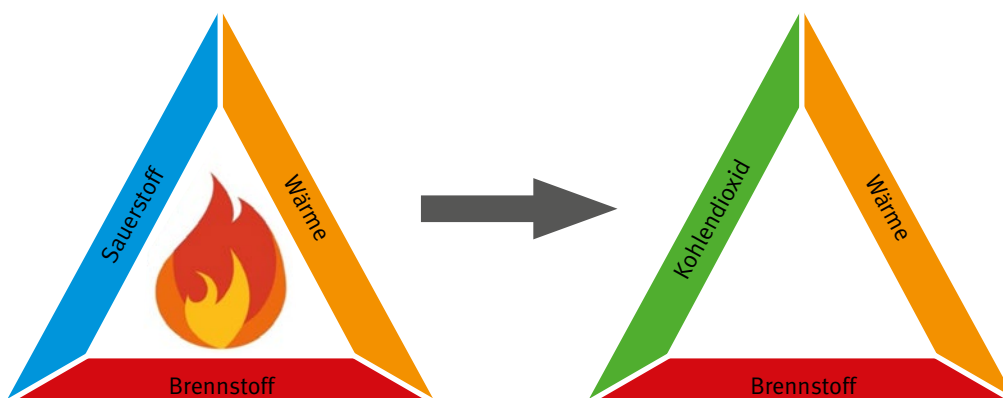
Abb. 7 Branddreieckdarstellungen unter Einflussnahme von Kohlendioxid (CO 2 ) auf das Erlöschen der Flamme
