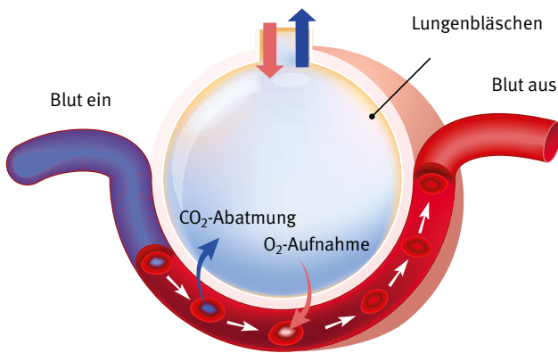
Abb. 6 Sauerstoff(O 2 )- und Kohlendioxid(CO 2 )-austausch in den Lungenbläschen
