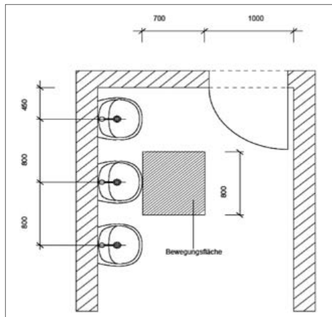
Abb.9.2 Waschaum (Maße in mm) nach ASR A4.1
