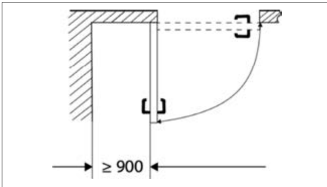
Abb. 3.4 Vermeidung von Quetschgefährdung bei kraftbetätigten Dreh- und Faltflügeltüren oder -toren (Maße in mm) (Quelle: ASR V3a.2)
