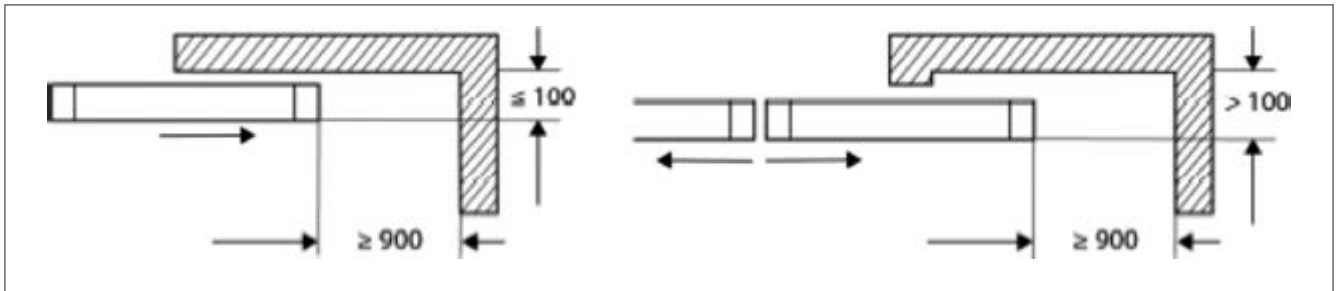
Abb. 3.3 Vermeidung von Quetschgefährdung bei kraftbetätigten Schiebetüren/-toren (Maße in mm) (Quelle: ASR V 3a.2)
