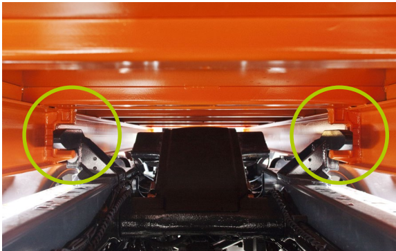
Abb. 39 Abrollbehälter ist über Verriegelungsdorn / Verrie- gelungsöse formschlüssig gesichert
