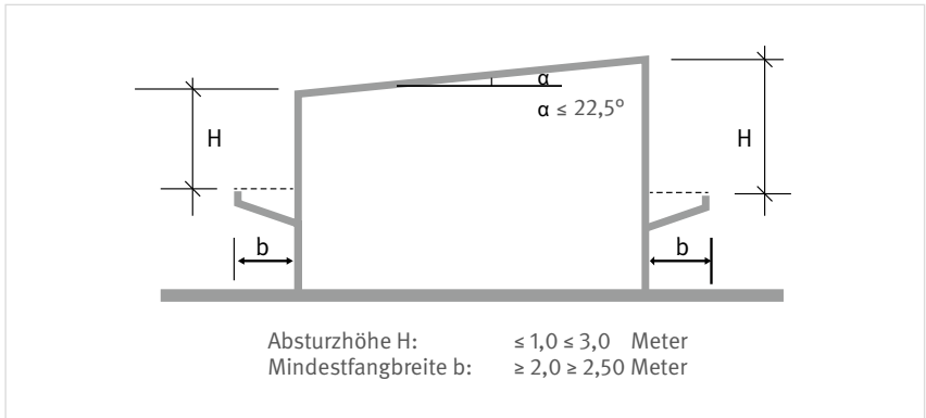
Abb. 11 Absturzhöhen der Schutznetze und erforderliche Fangbreiten bei 0° bis 22,5° geneigten Flächen
