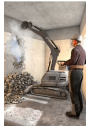
Abb. 32 ferngesteuertes Abbruchgerät
